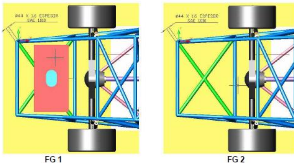
Montaje y ubicación de tanques de combustible: FG 1 Y 2
